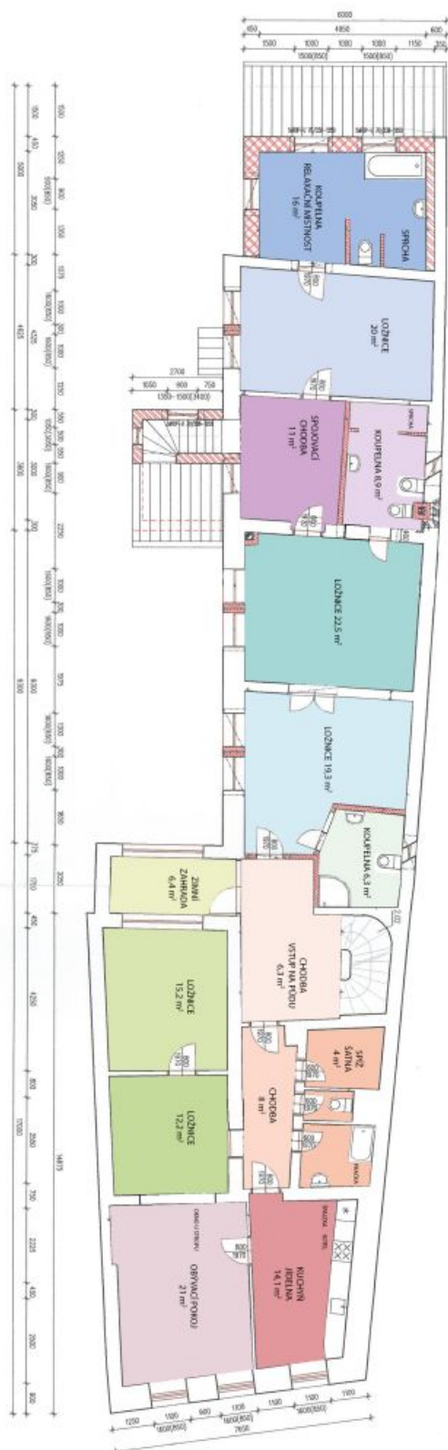
HUSOVA 32, PŮDORYS 2. NADZEMNÍ PODLAŽÍ
