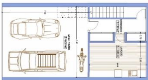
PLANTA SOTANO
