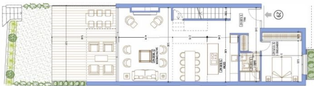
PLANTA BAJA
