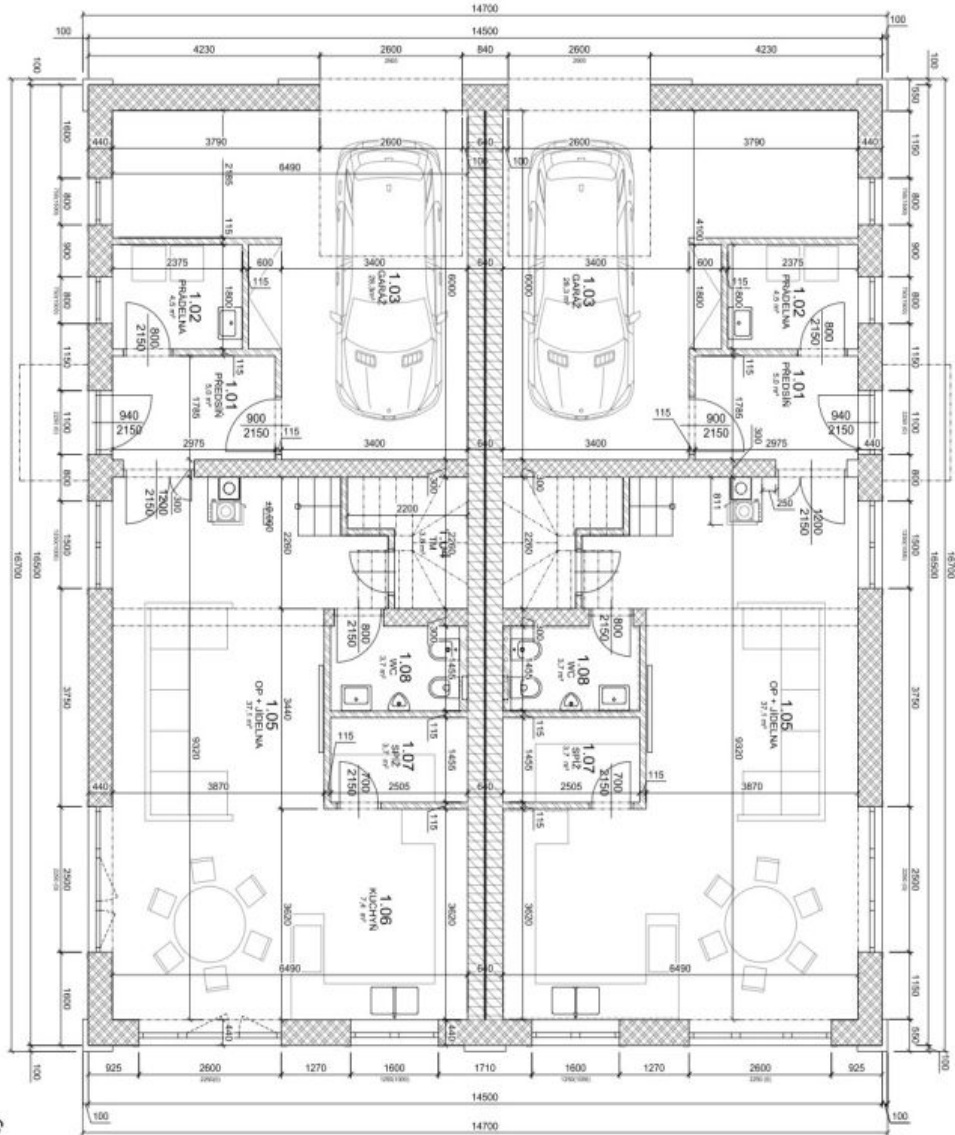
PŮDORYS 1 NADZEMNÍHO PODLAŽÍ
