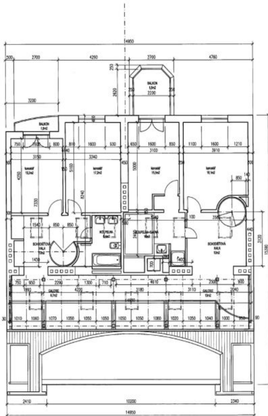
Půdorys 6.NP
