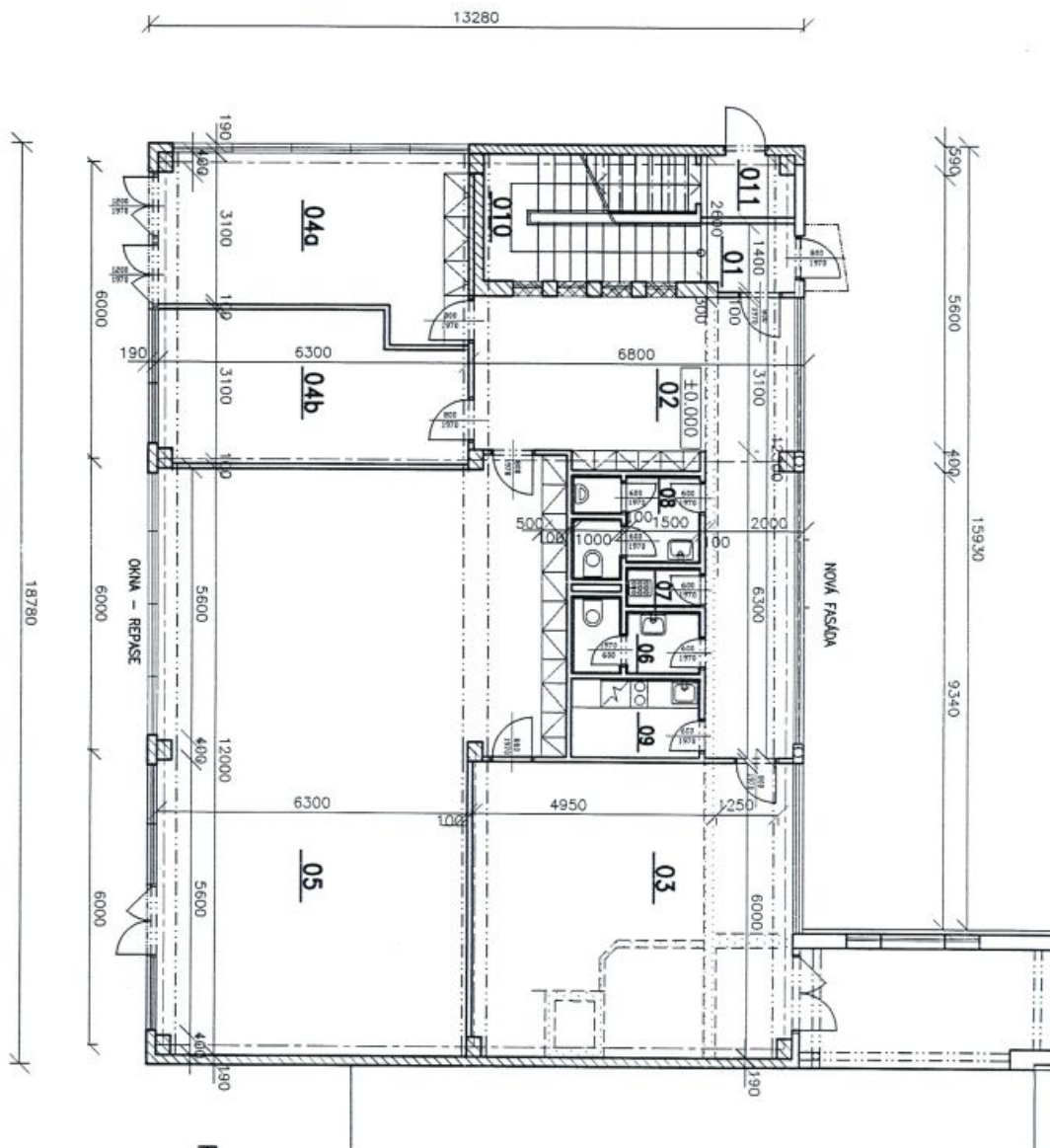
PŮDORYS 1.NP
