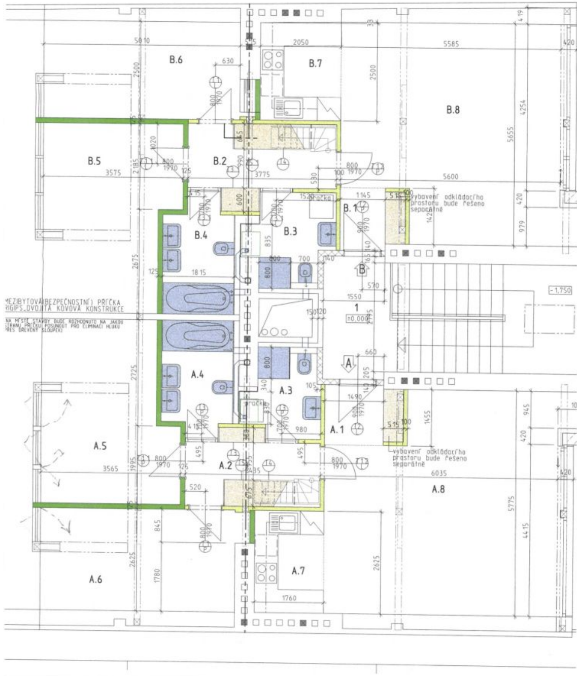
1RYS PODKROVÍ, 1/50
