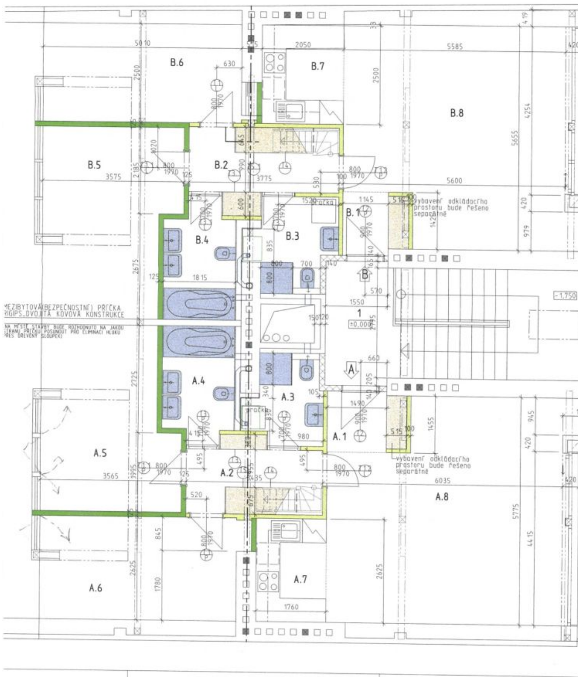
1RYS PODKROVÍ, 1/50
