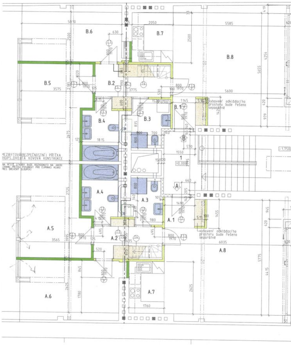
1RYS PODKROVÍ, 1/50
