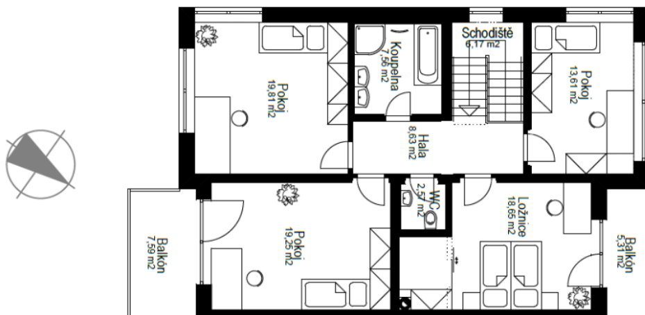
PŮDORYS 2.NP
