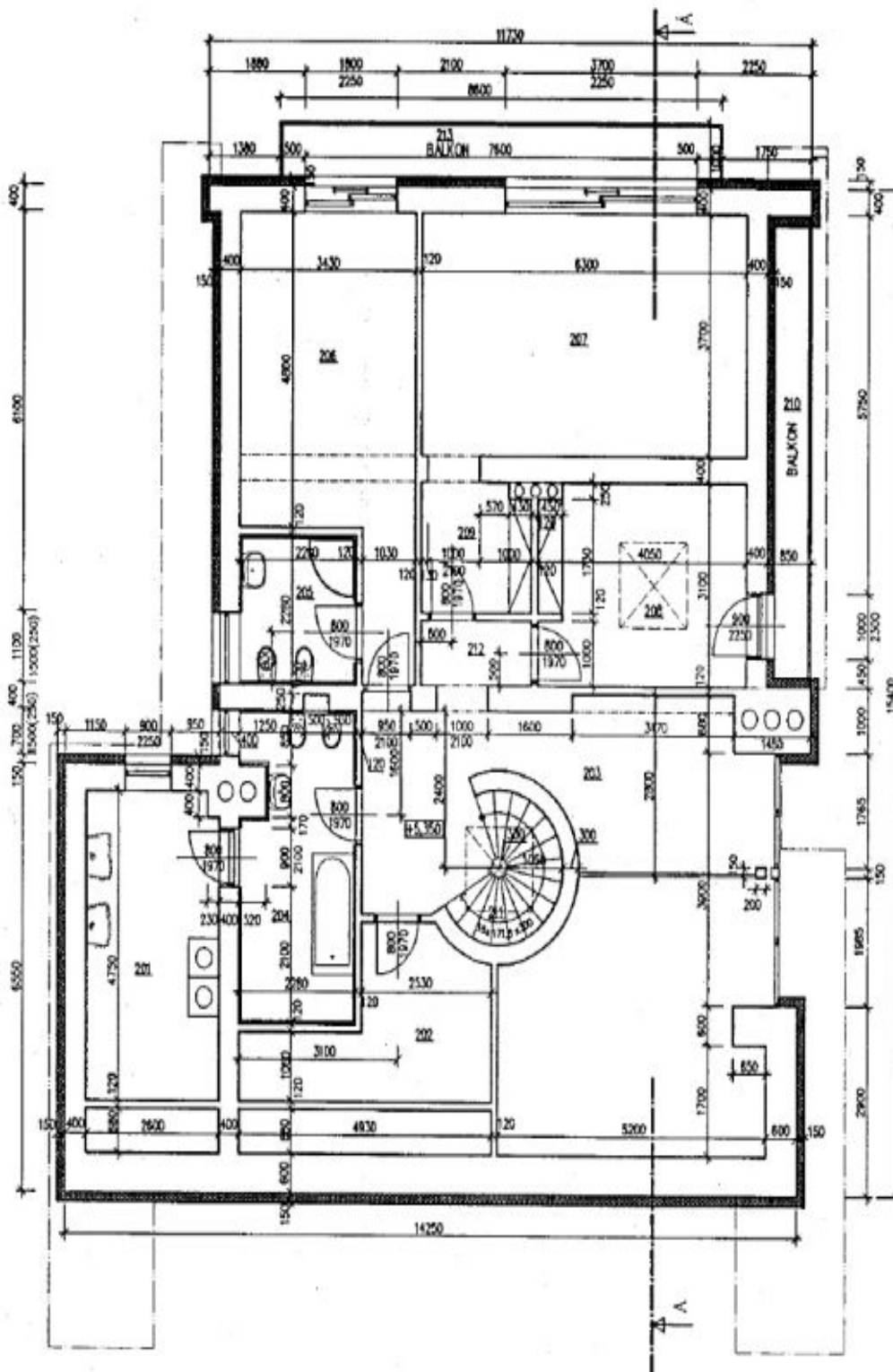
PŮDORYS 2.NP
