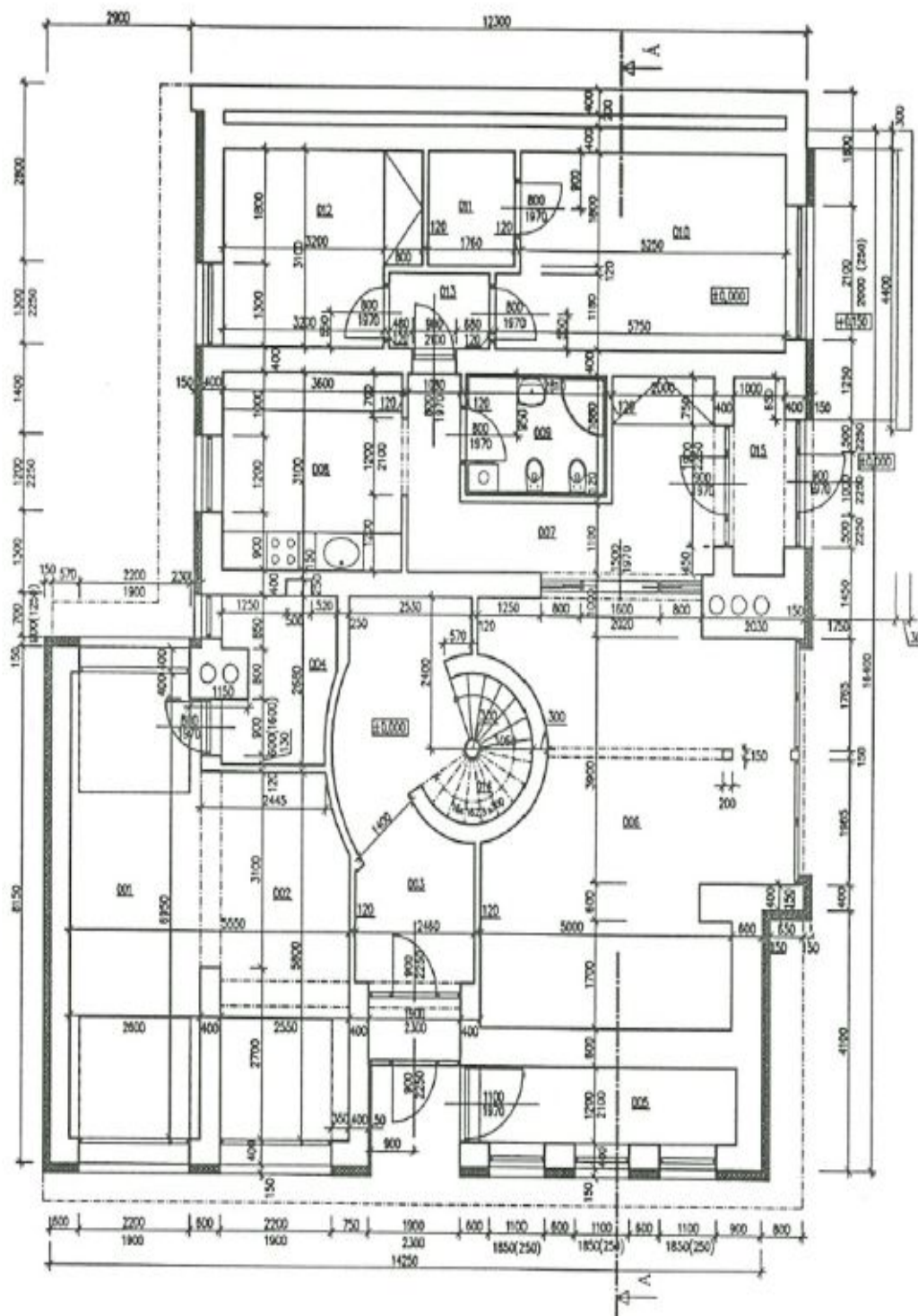
PŮDORYS I.PP
