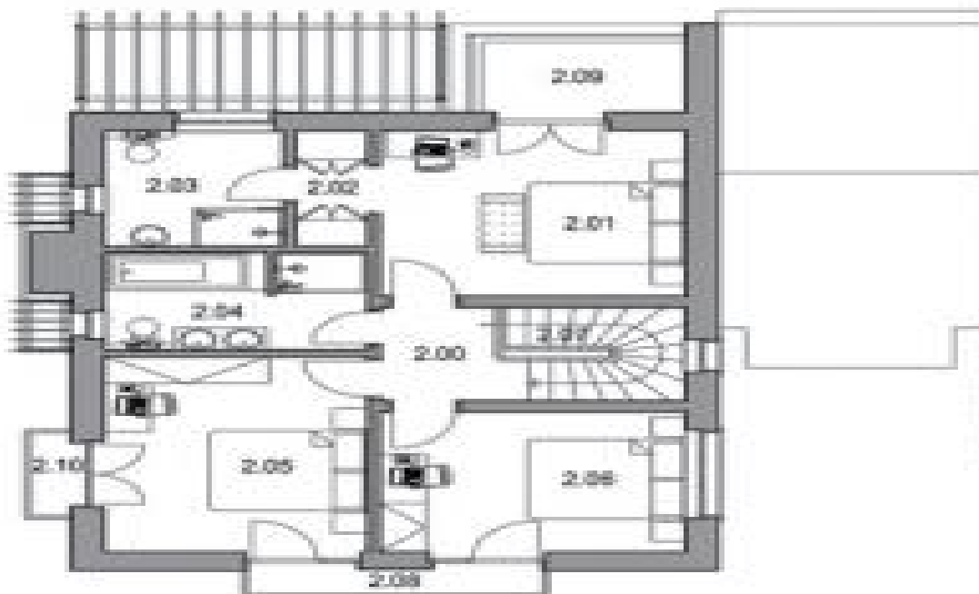
PŮDORYS 2.NP / FIRST FLOOR
