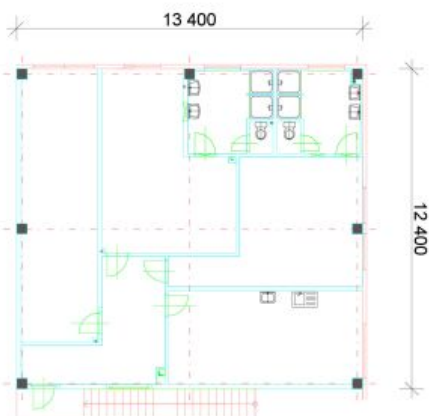
PŮDORYS 2.NP
