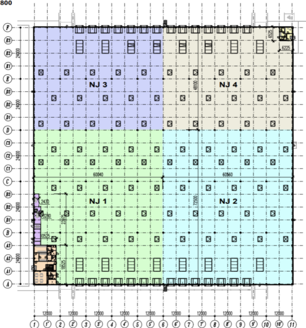
PŮDORYS 1.NP 1:800
