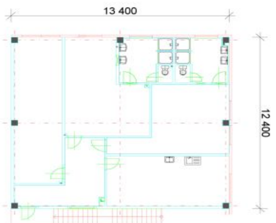
PŮDORYS 2.NP
