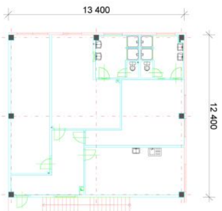
PŮDORYS 2.NP
