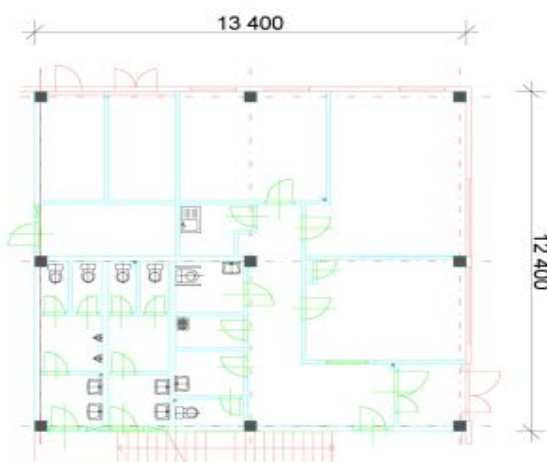
PŮDORYS 1.NP
