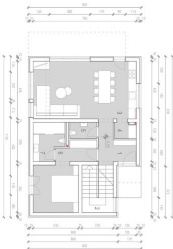
TLOCRT PRIZEMLJA
